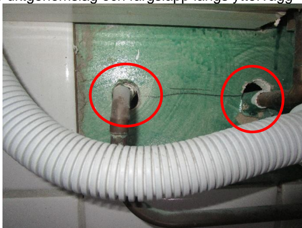
Otåta rörgenomföringar i vägg under handfat
