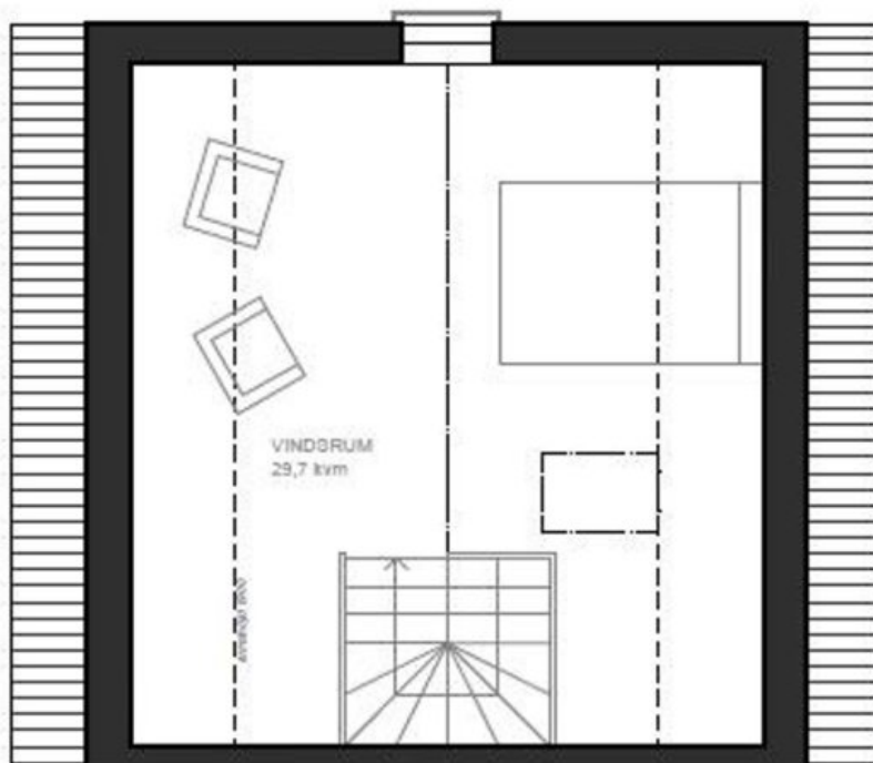
PLAN 3 vind
