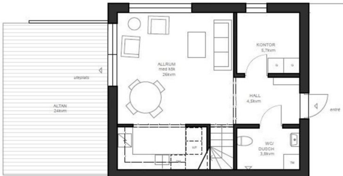
PLAN 1 marknivå
