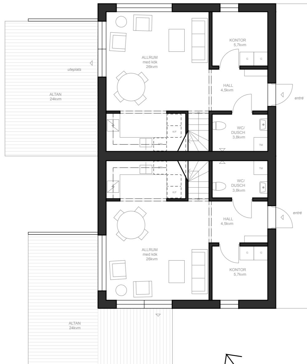
PLAN 1 marknivå
