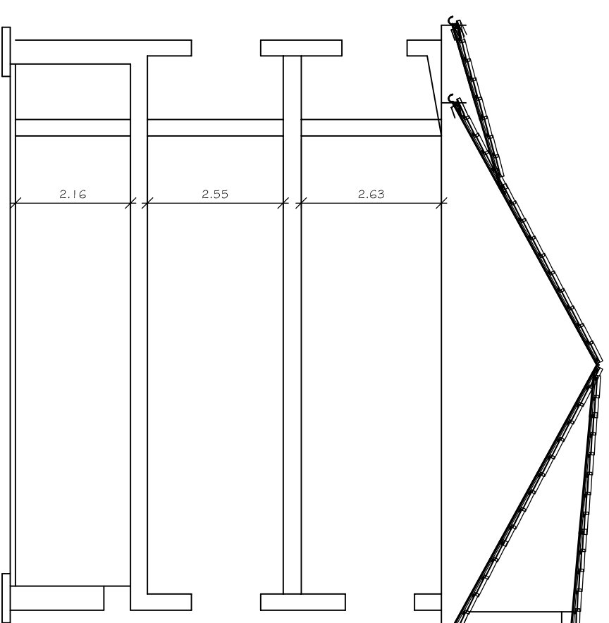
SEKTION
